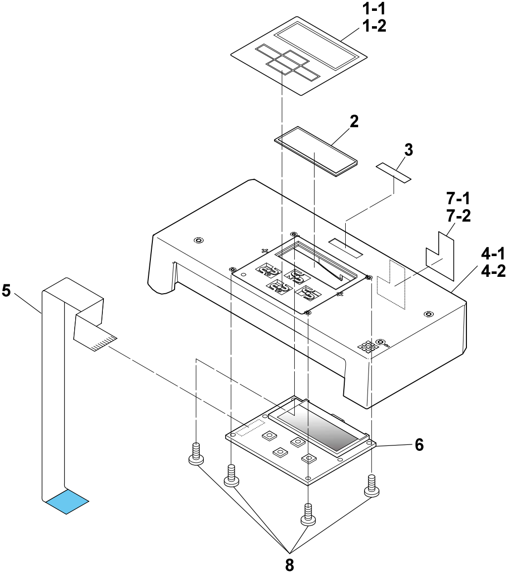
DRAWING NO. 8 SA Cover (Rev. 0)
