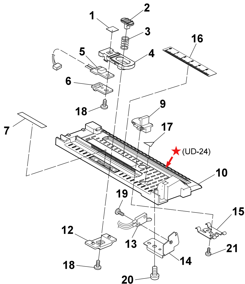
DRAWING NO. 6 SA Guide Paper L (Rev. 0)
