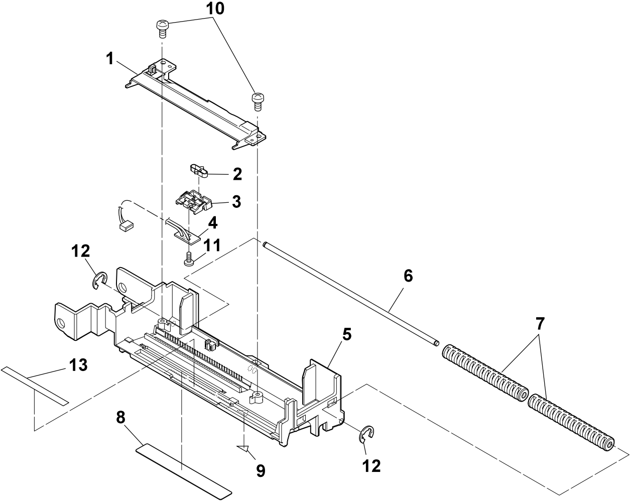
DRAWING NO. 5 SA Guide Paper U (Rev. 0)
